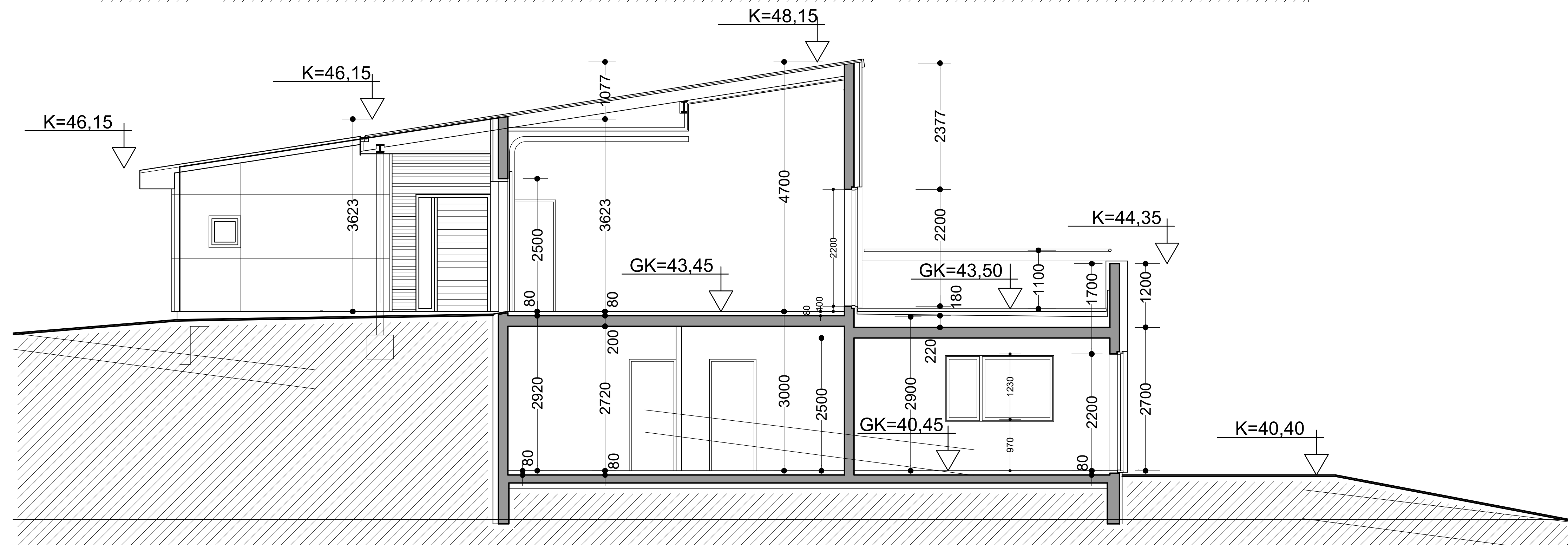
Snið B-B mkv. 1:50
