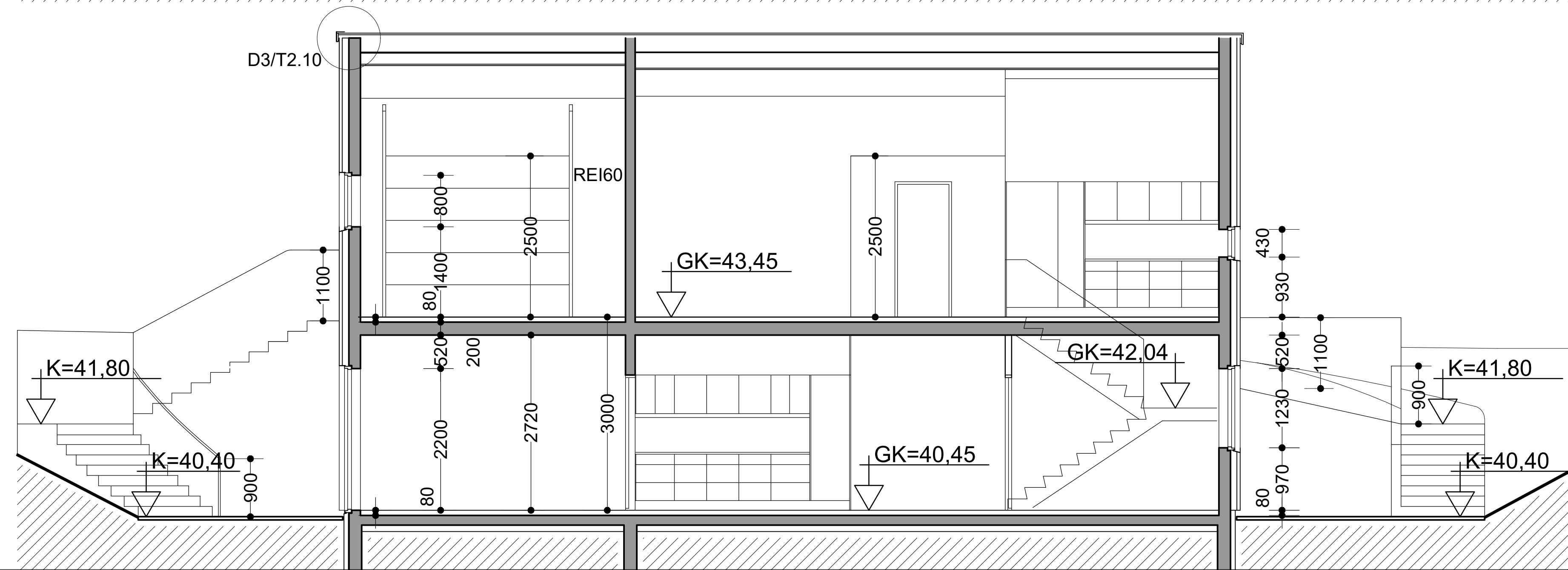
Snið C-C mkv. 1:50
